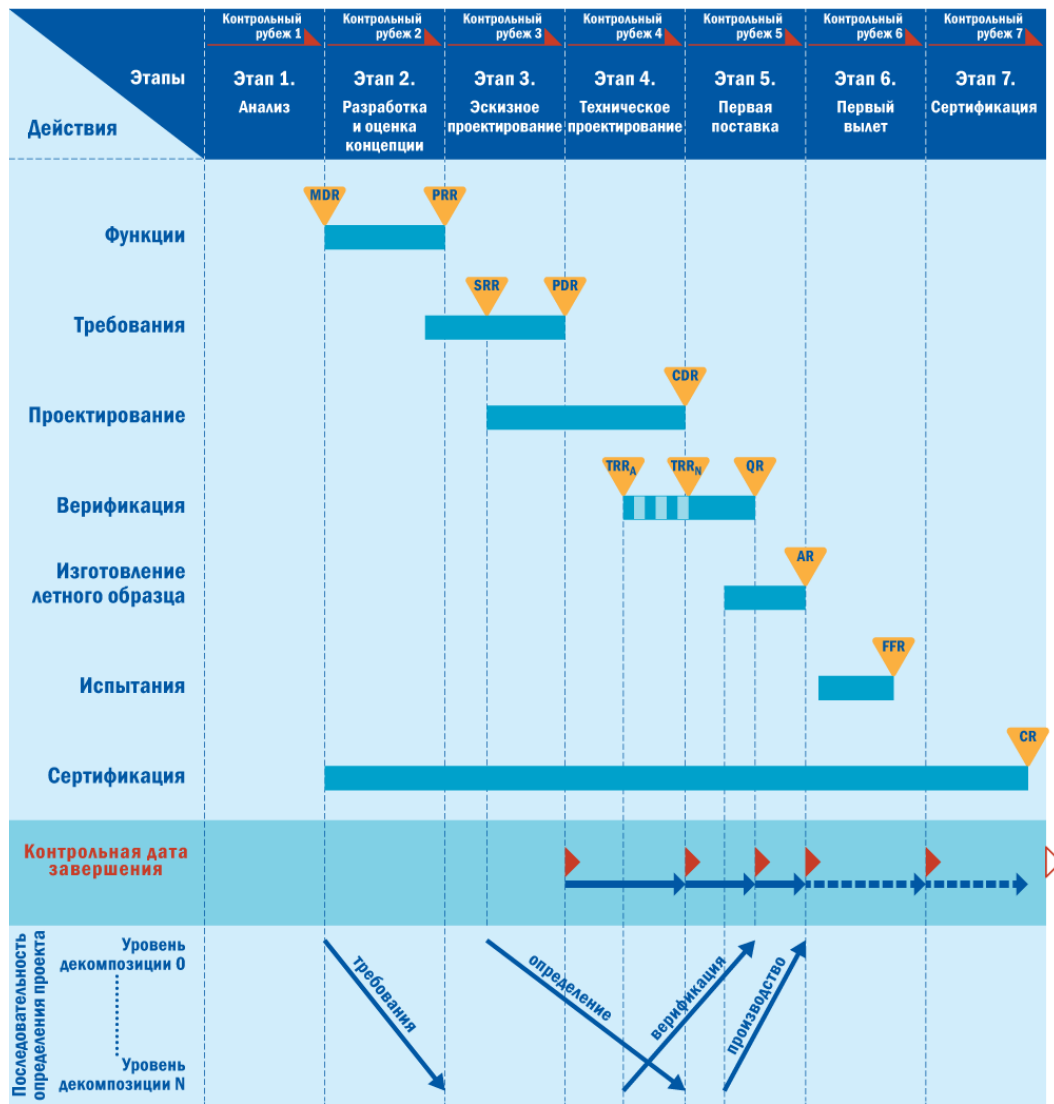
Рис. 1.9. Связь ТЭ КБО на уровне ВС с процессами и этапами разработки ВС.
