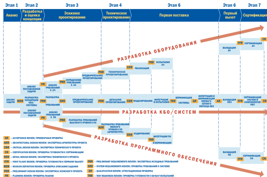
Рис. 1.8. Технические экспертизы (ТЭ) процессов разработки КБО, систем и компонентов.
